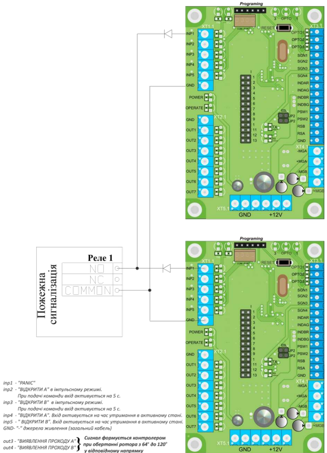
Додаток Г.4. Схема електричного підключення турнікетів до пожежної сигналізації (ПС)
