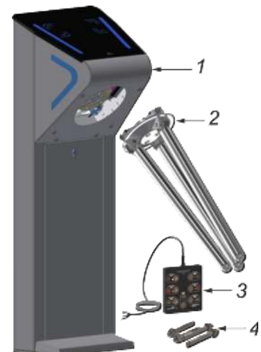
Рис. 3 – Комплект поставки турнікета-трипода
